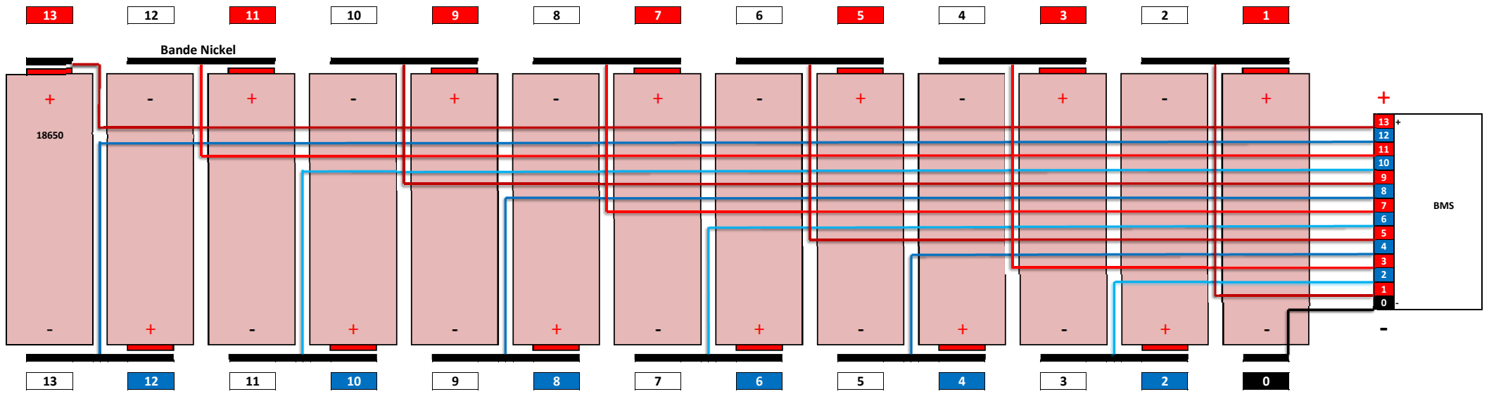
Pack Batterie 18650 13S - Connexion BMS
